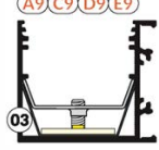
VARIO30-03
