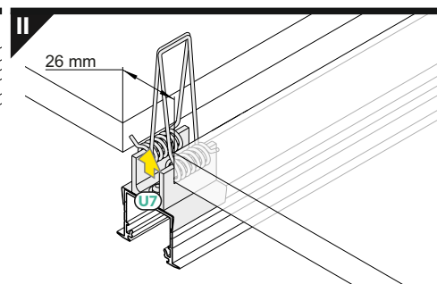
držák U7, otvor zahluobený cone U7 mounting plate
