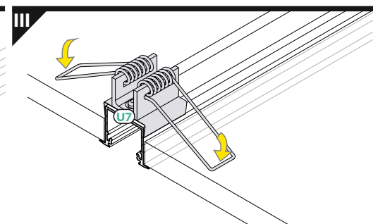
držák U7 rozpěrný se zuby do drážky rack U7 mounting plate
