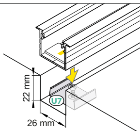
držák U7, otvor zahluobený cone U7 mounting plate
