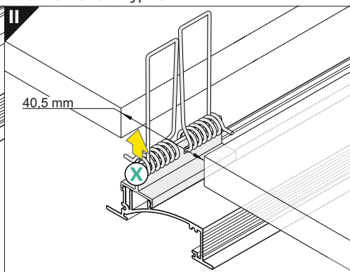
držák U pružný, otvor zahlbouný cone U flexible mounting plate
