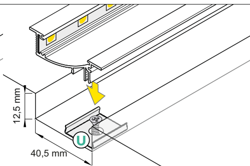
držák U pružný, otvor zahlbouný cone U flexible mounting plate
