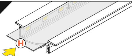
difuzor H nasouvací / H slide cover
